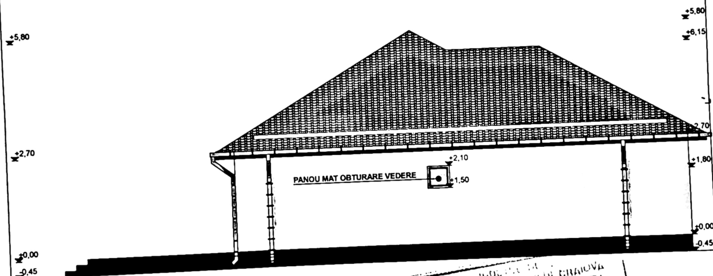
FATADA SUD
